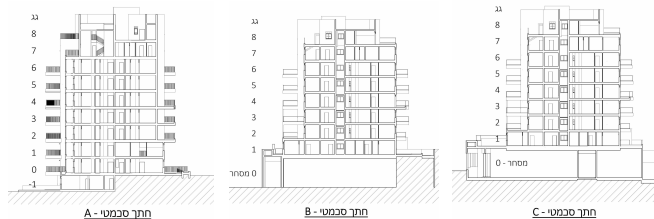
חתכים סכמטיים
